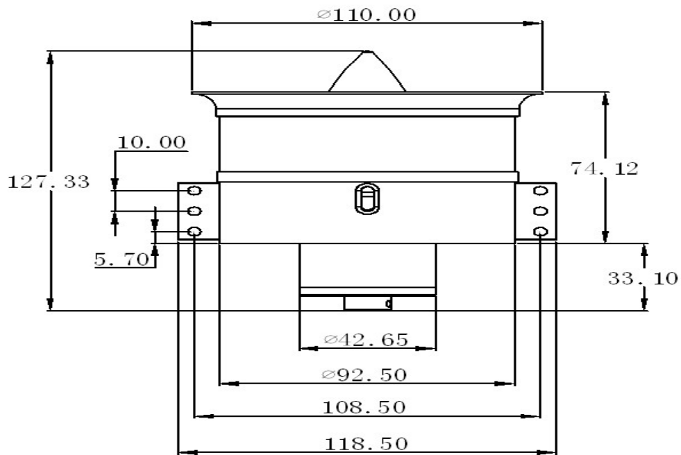
尺寸图 dimensional drawing(mm)
